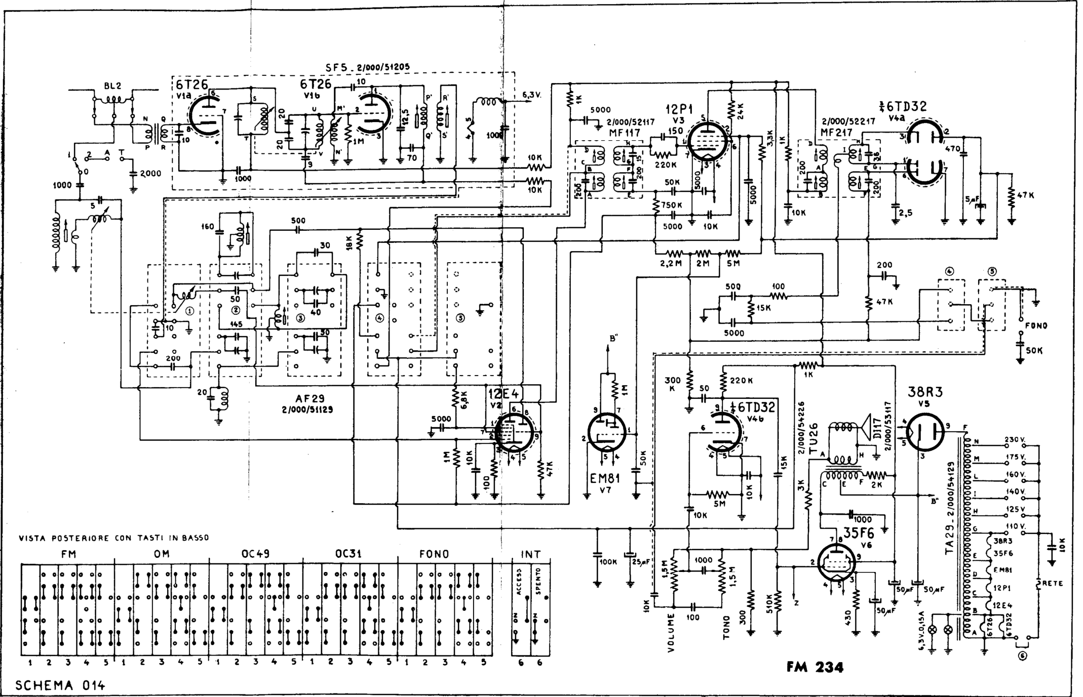
RAYMOND (GARUFI) - Mod. FM 234. Apparecchio AM/FM con una gamma onde medie da 520 a 1620 kc/s, una banda allargata ad onde corte a 49 metri ed una seconda banda allargata a 31 metri. Banda ad onde ultracorte a modulazione di frequenza. Media frequenza AM a 471 kc/s, media frequenza FM a 10,7 Mc/s. Commutazione a tasti. Potenza d'uscita 4 watt. Assorbimento 50 watt.
